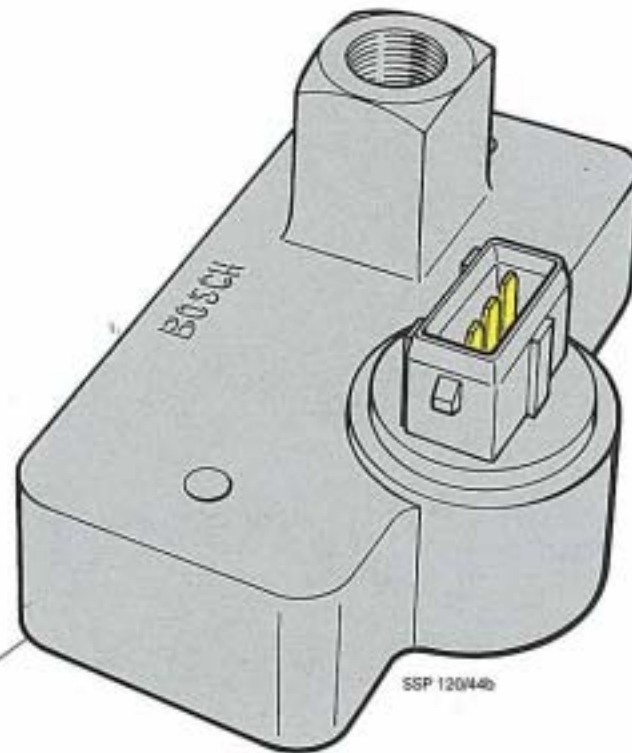
Ladedruckfühler
